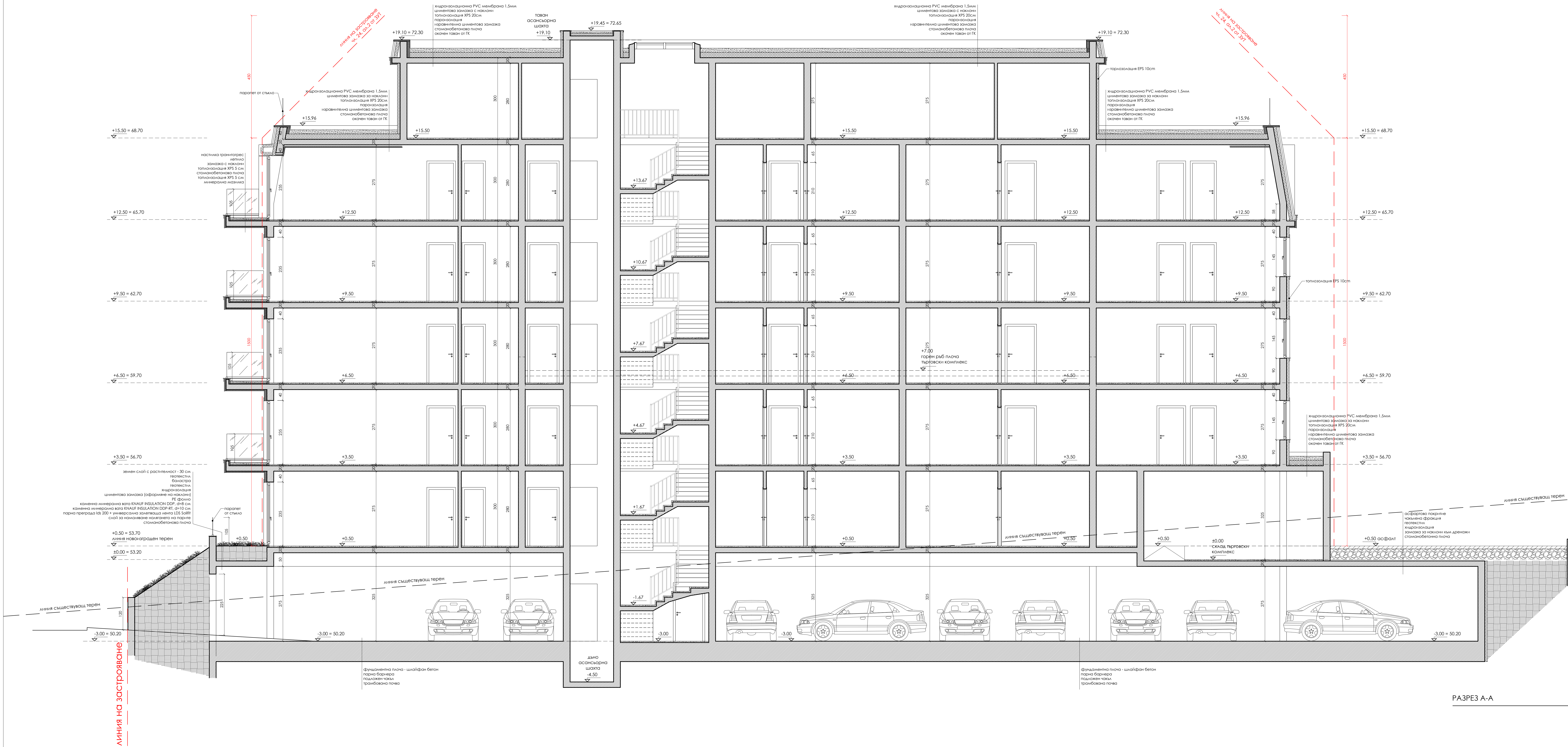
PA3PE3 A-A M 1:50
