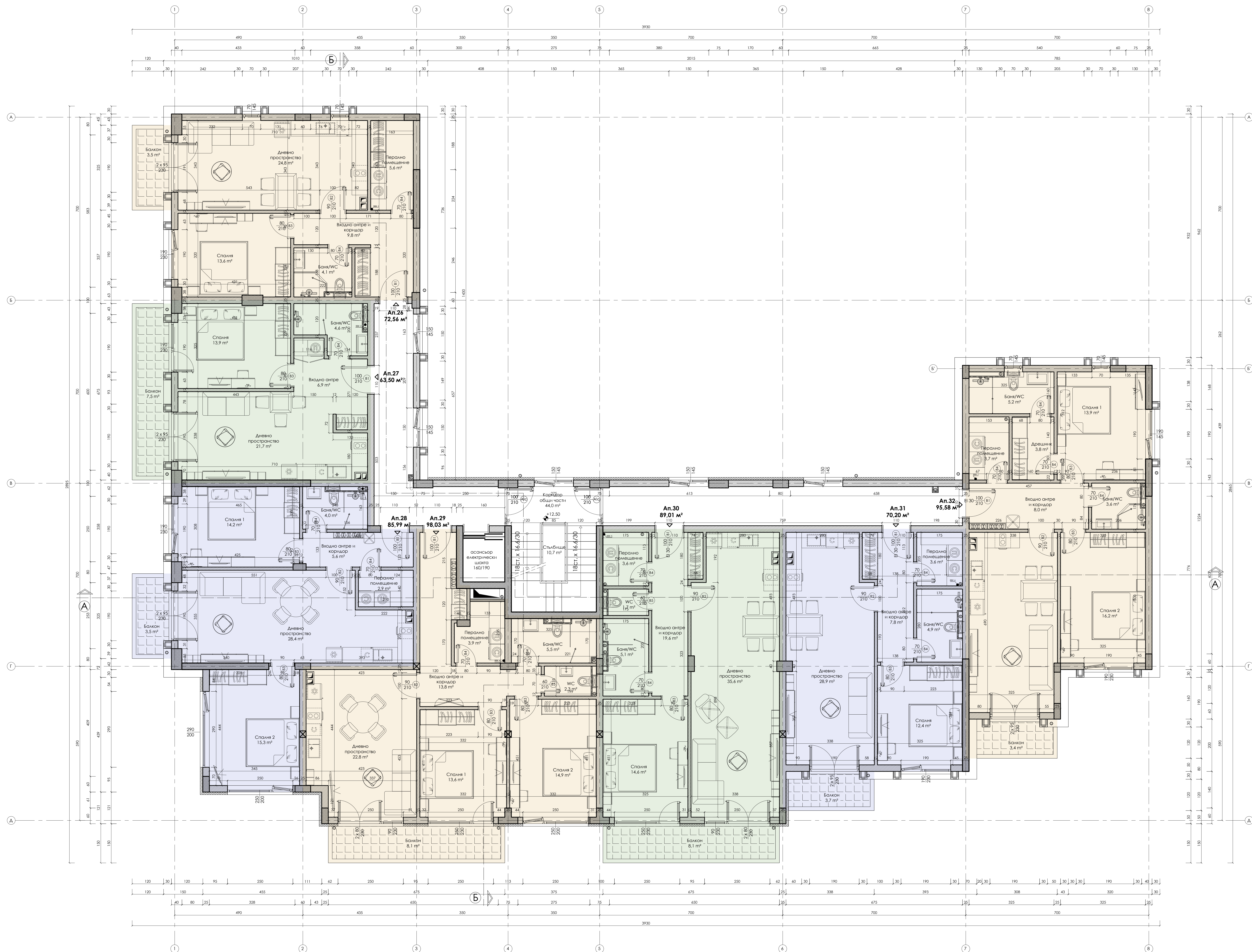
РАЗПРЕДЕЛЕНИЕ НА КОТА +12.50 (ПЕТИ ЕТАЖ) ЗП 656,9 м²
