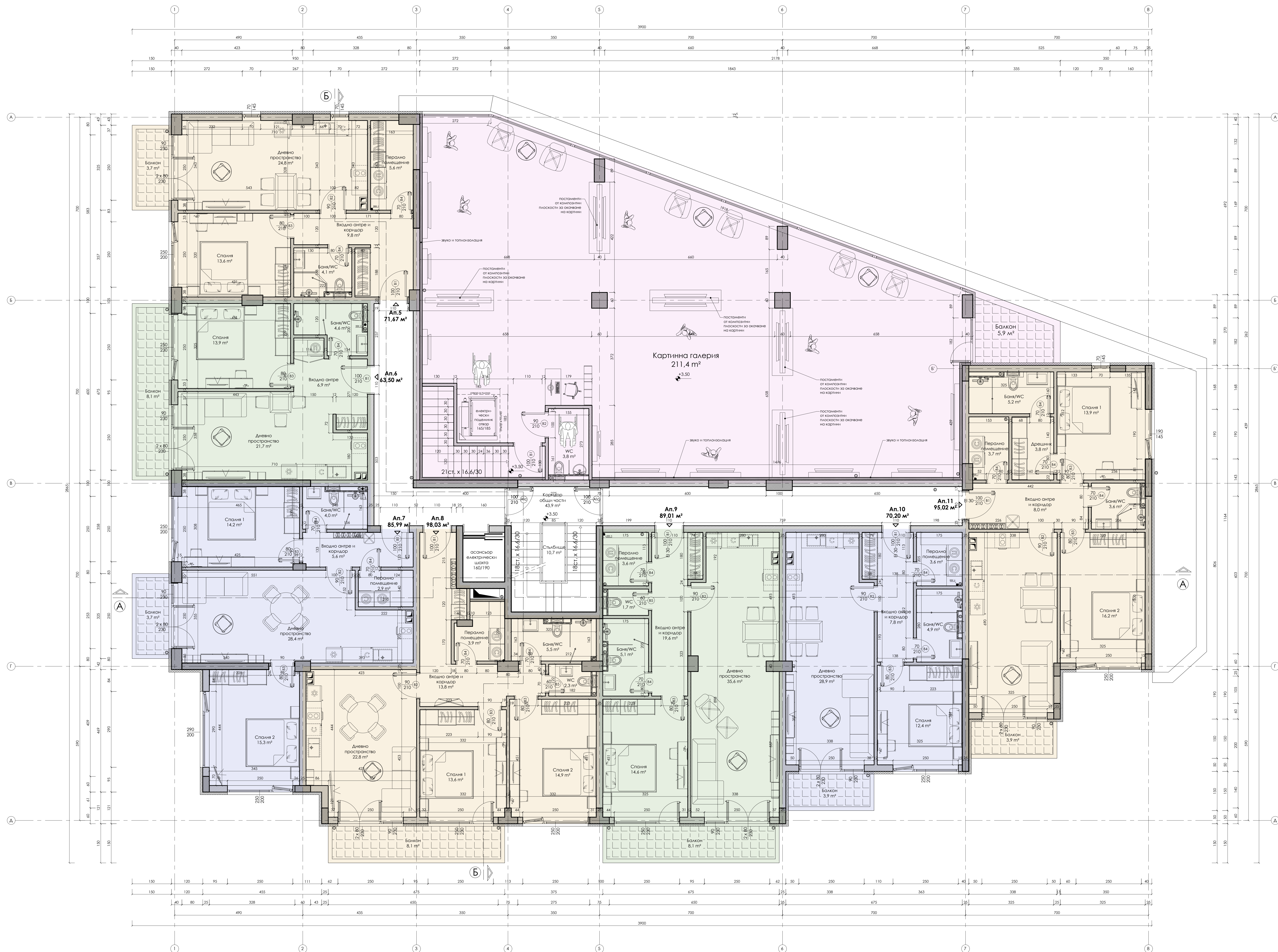
РАЗПРЕДЕЛЕНИЕ НА КОТА +3.50 (ВТОРИ ЕТАЖ) ЗП 894,2 м²
