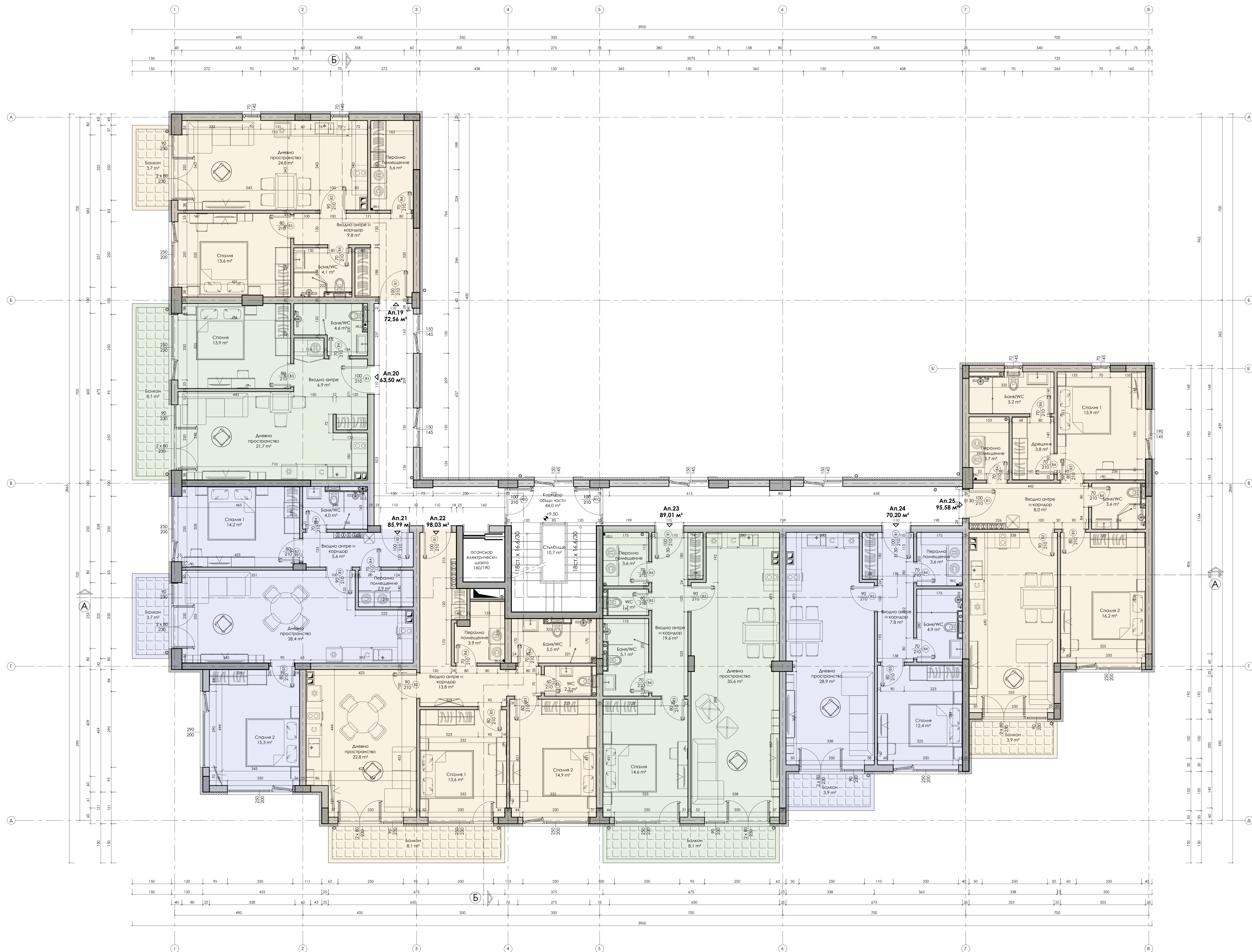
РАЗПРЕДЕЛЕНИЕ НА КОТА +9.50 (ЧЕТВЪРТИ ЕТАЖ) ЗП 656,9 м 2
