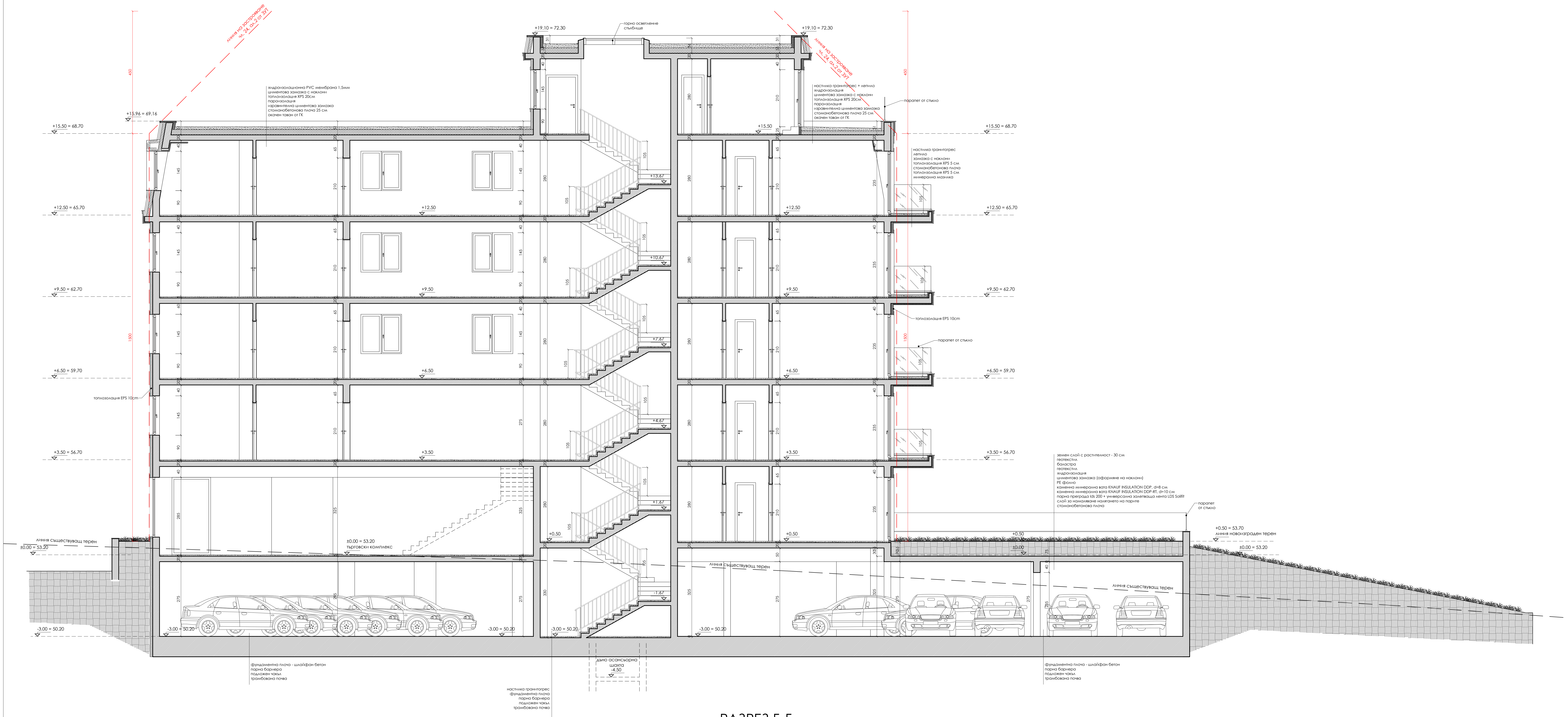
РАЗРЕЗ Б-Б М 1:50
