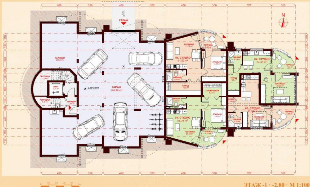
ЭТАЖ -1 • -2,80 • М 1:100
