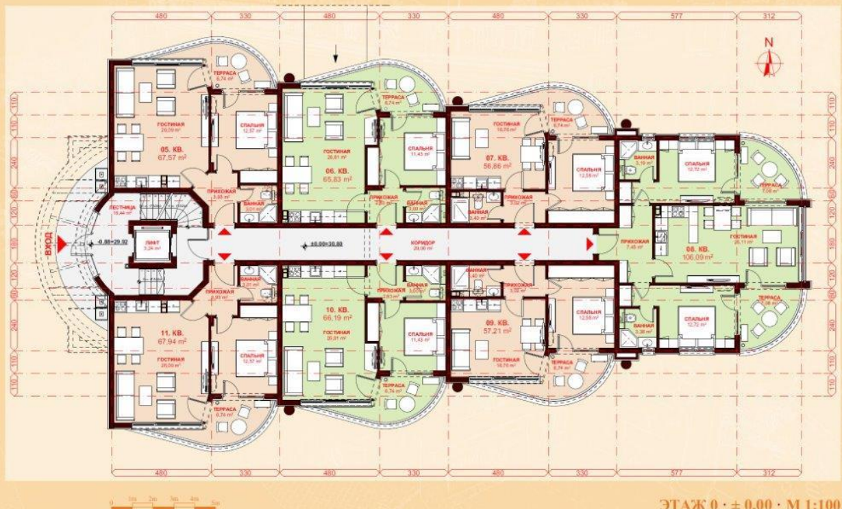
ЭТАЖ 0 • ± 0,00 • М 1:100
