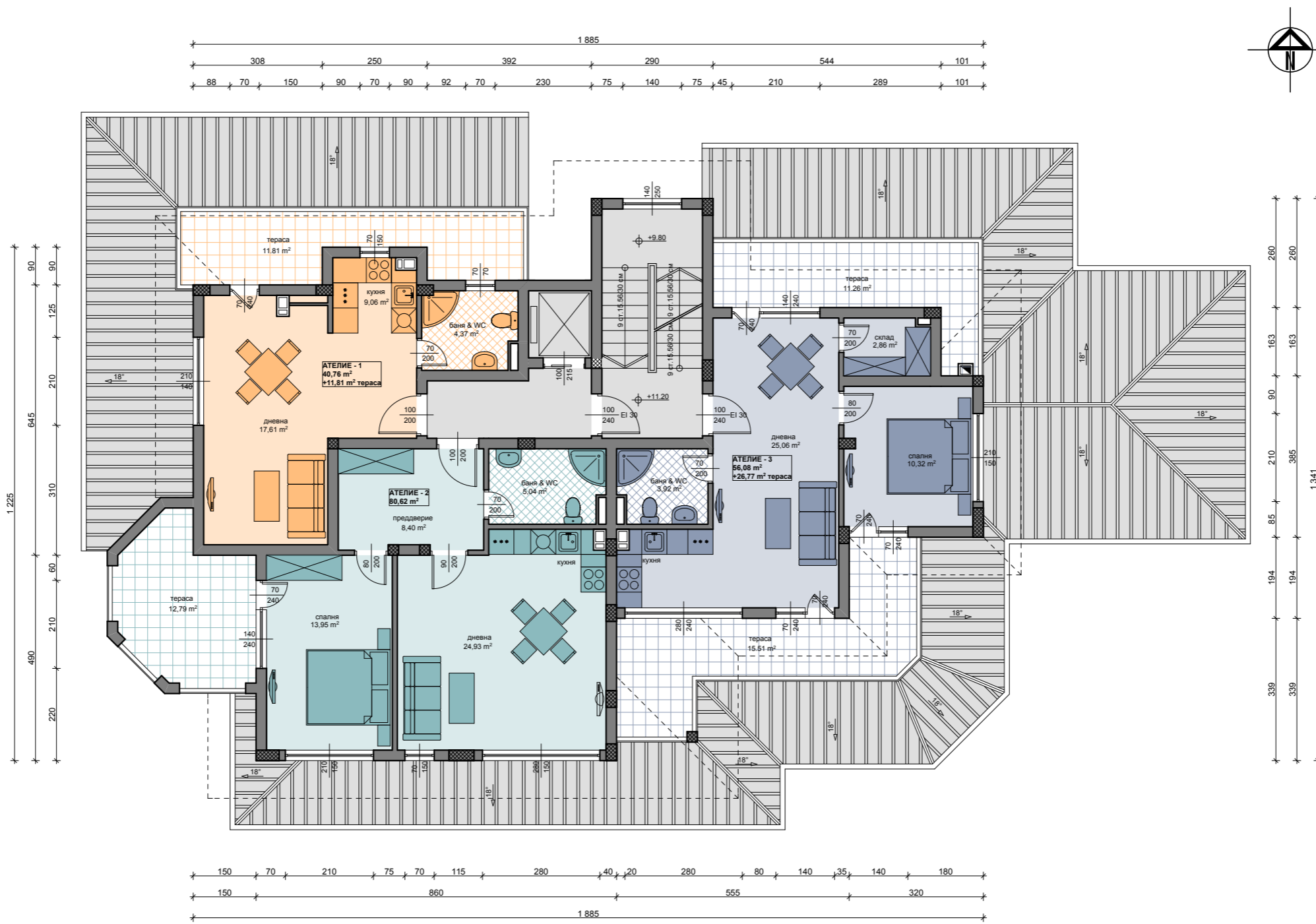
РАЗПРЕДЕЛЕНИЕ КОТА +11.20
