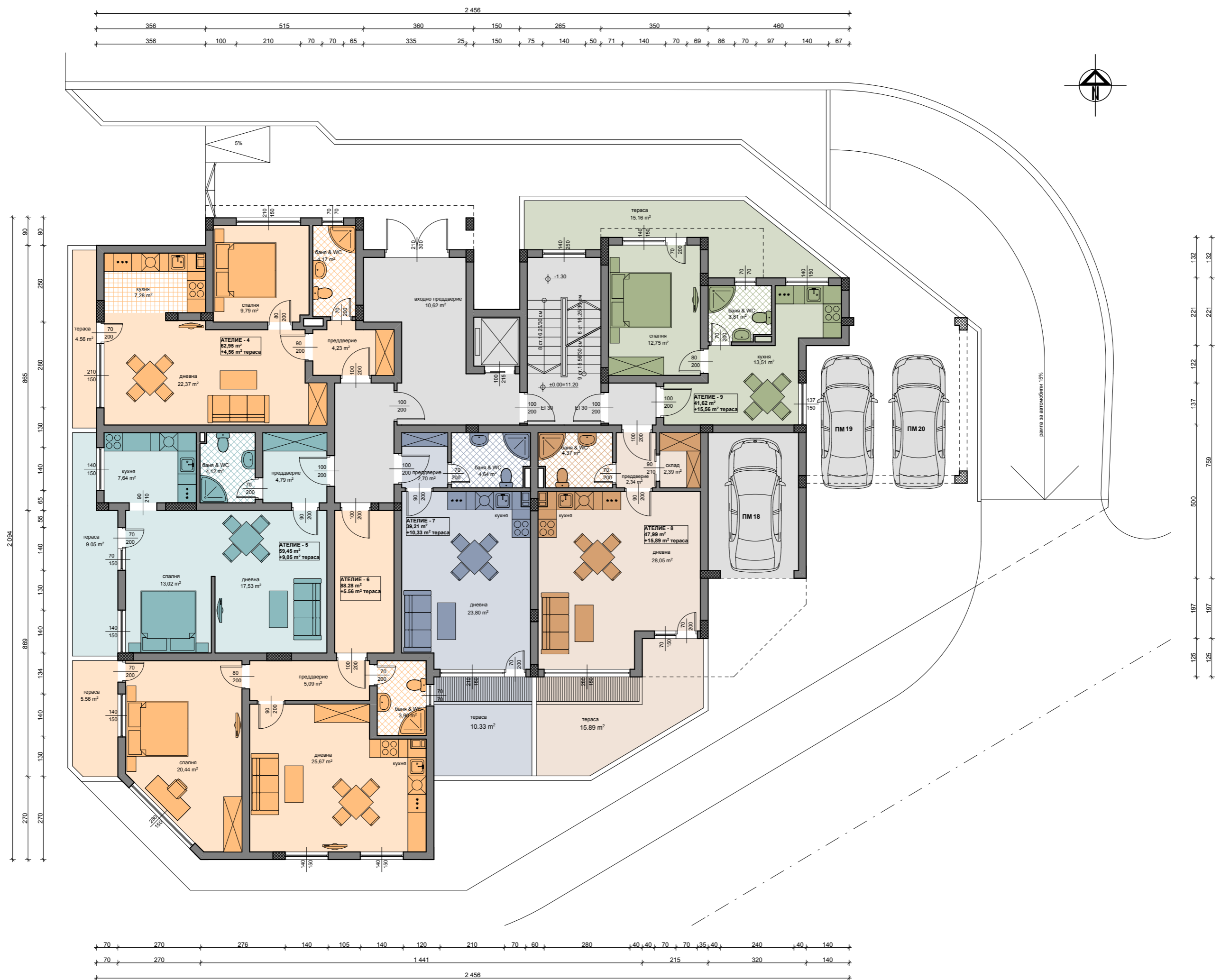
РАЗПРЕДЕЛЕНИЕ КОТА ±0.00
