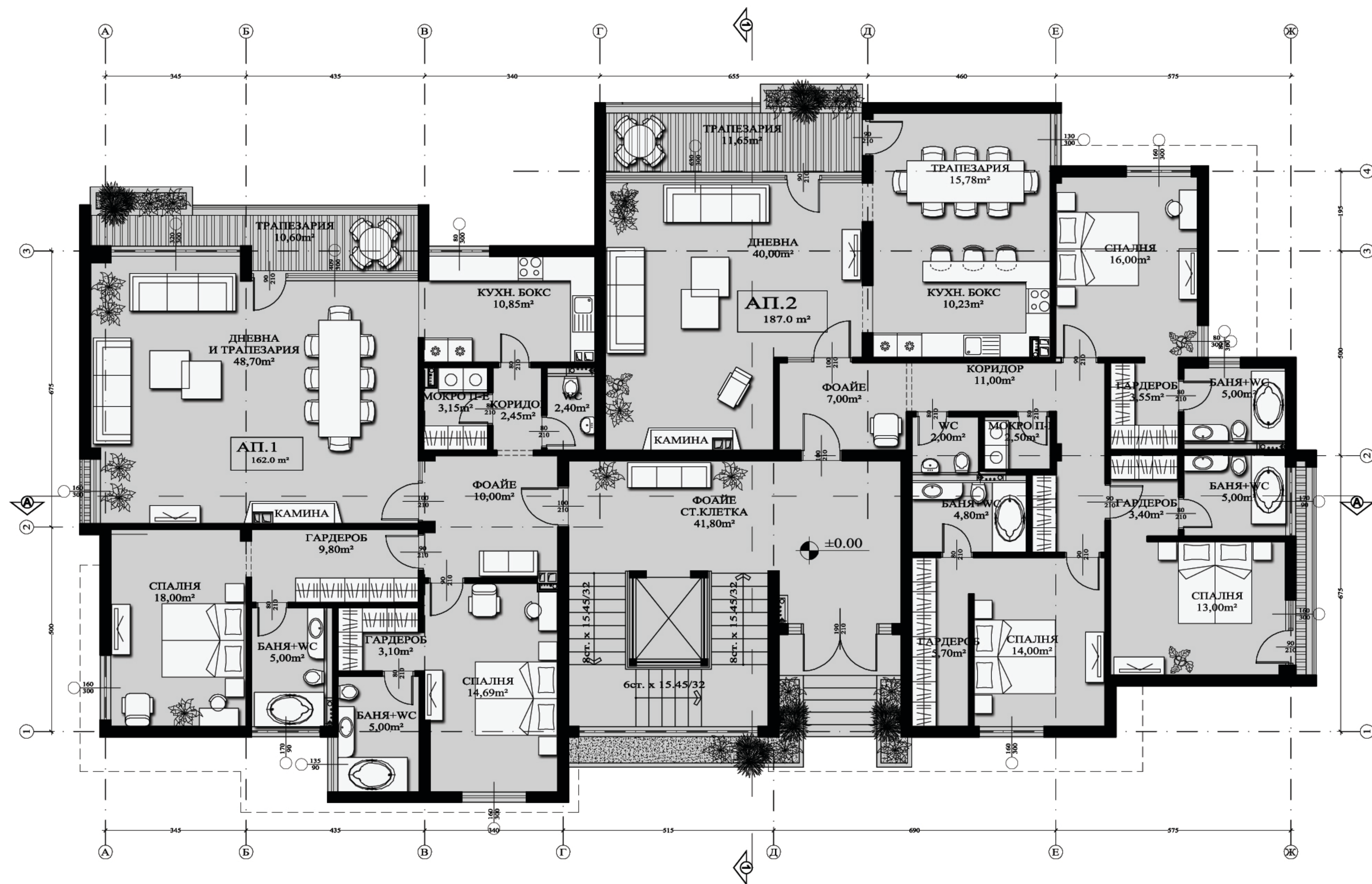
План Първи етаж ЗП - 404м2
