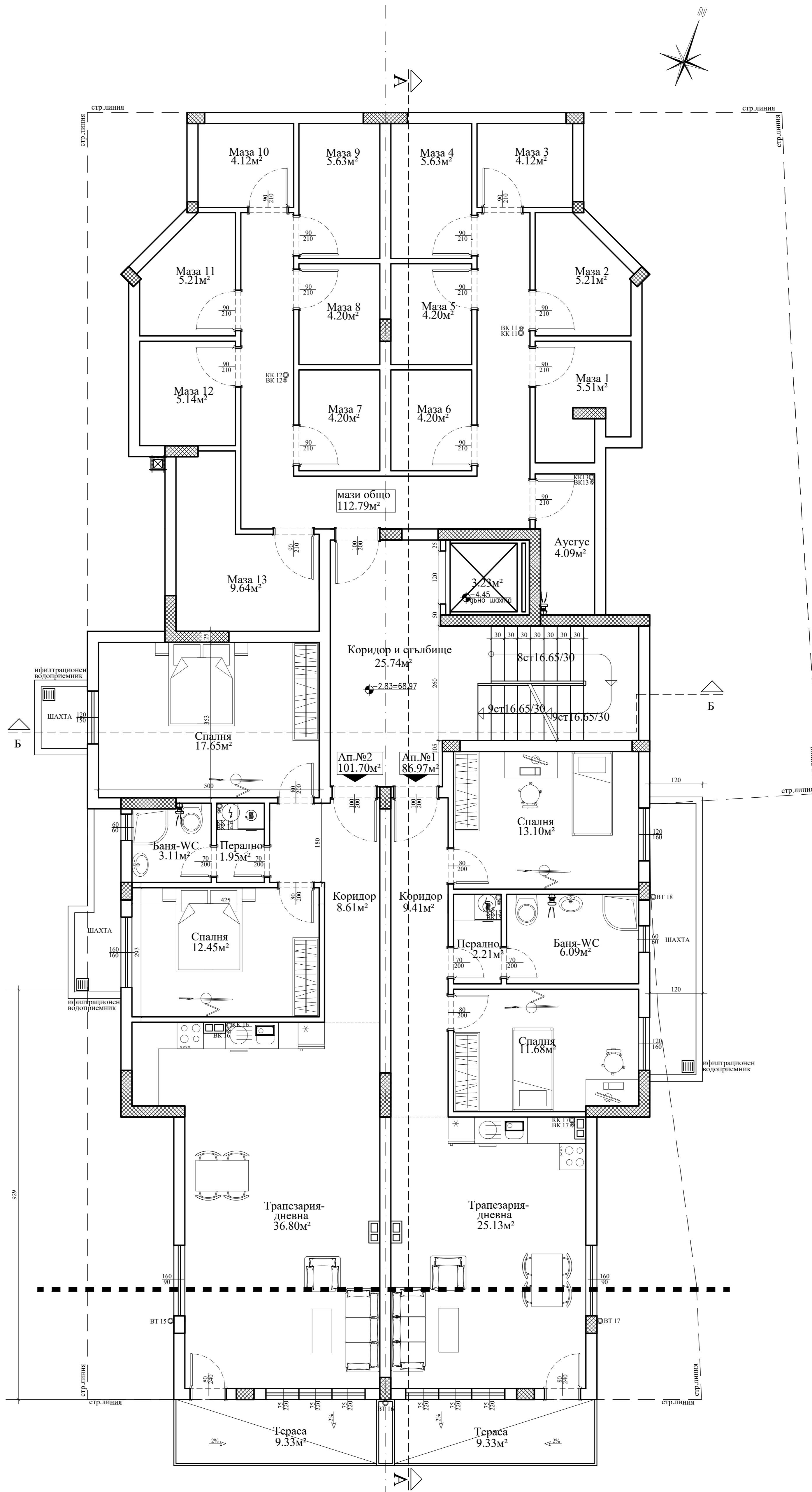
РАЗПРЕДЕЛЕНИЕ ПОЛУПОДЗЕМЕН ЕТАЖ КОТА -2.83
